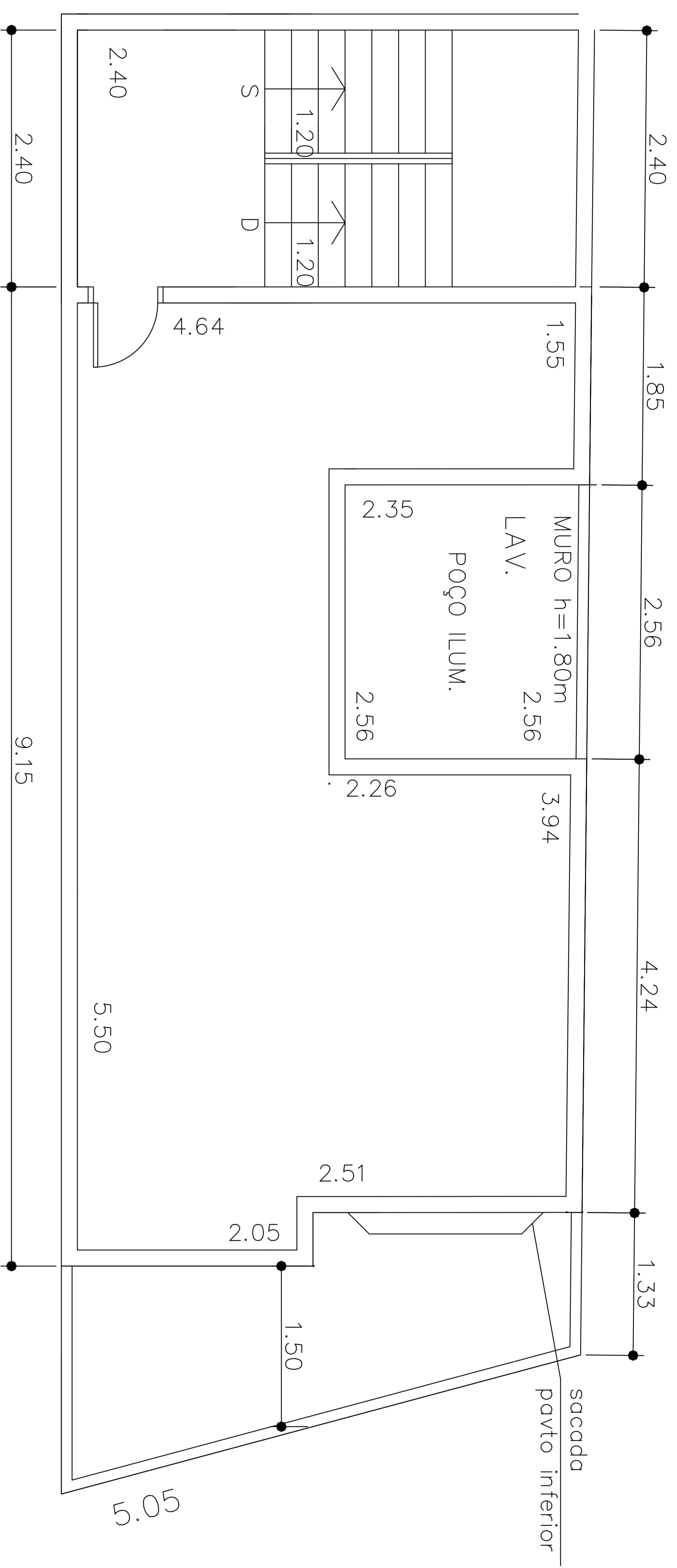
PLANTA DA UNIDADE DO FUNDO – COBERTURA
